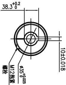
齿轮轴端面
