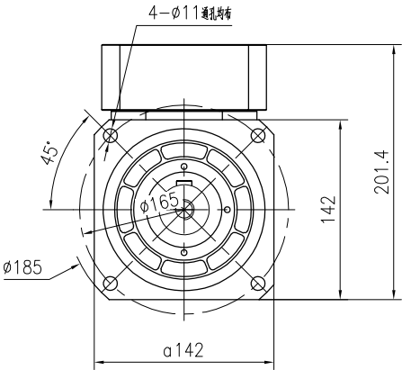
输出端(Output)
