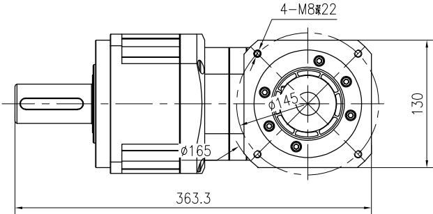
输入端
