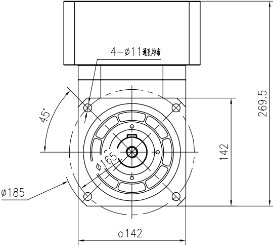
输出端(Output)
