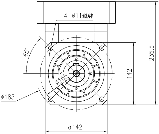
输出端(Output)
