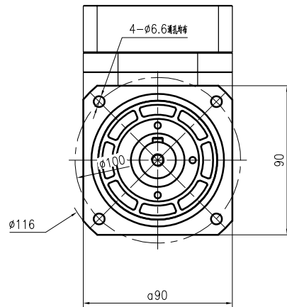
输出端(Output)
