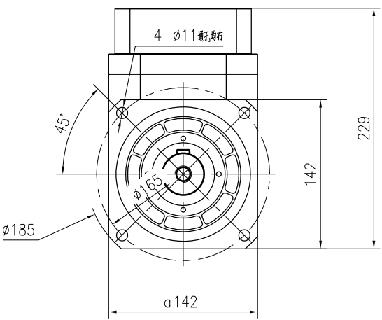
输出端(Output)
