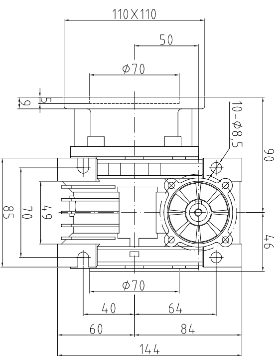
输出孔
