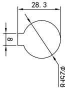
输出轴 细节A 比例2:1
