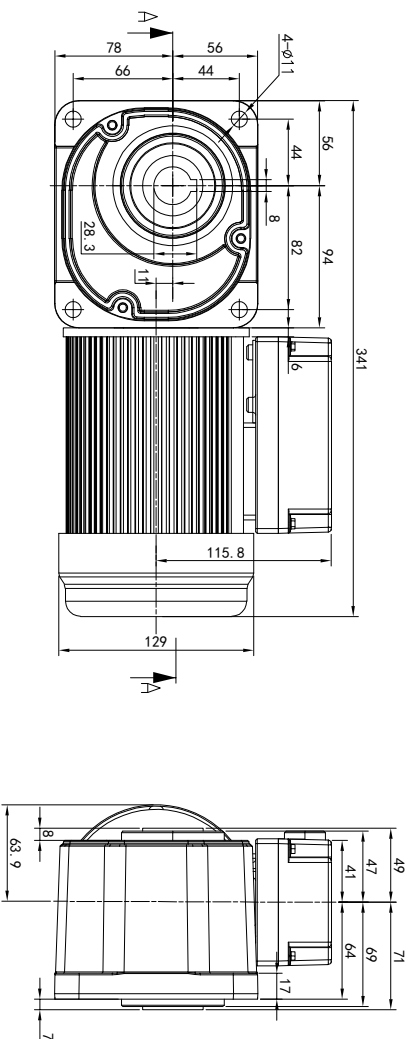
剖面 A-A
